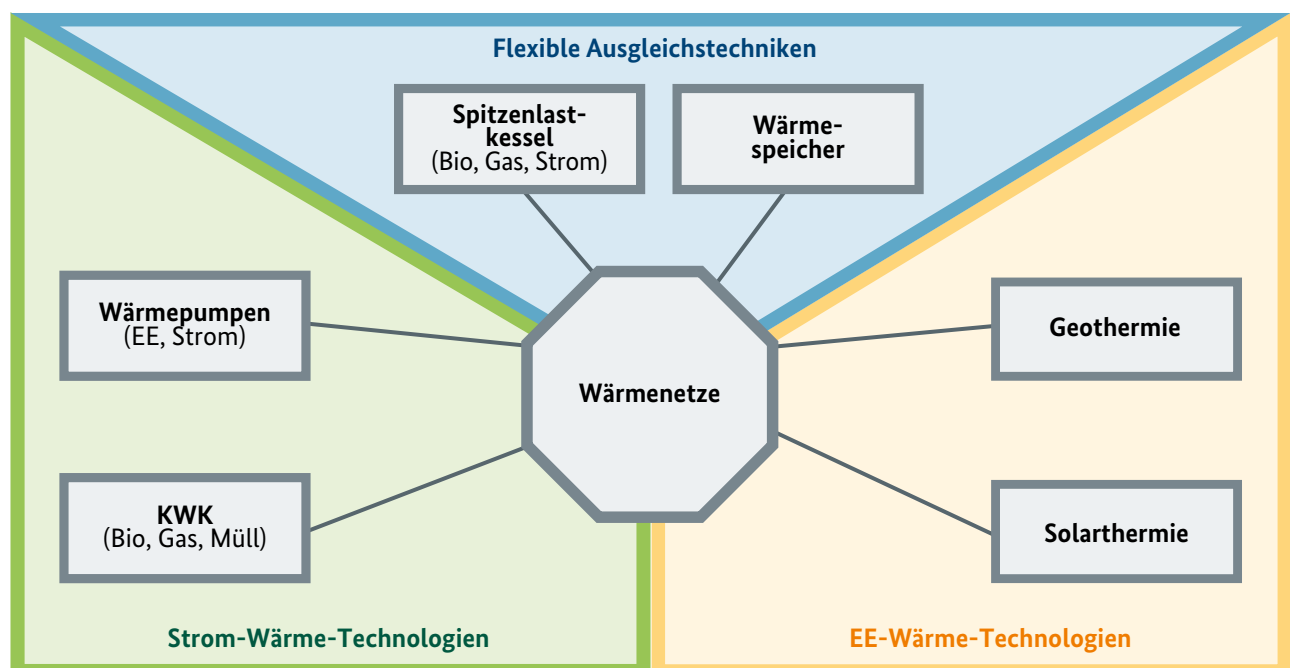
Abbildung 9: Modernes wärmenetzbasierendes Strom-Wärme-System (schematische Darstellung)
